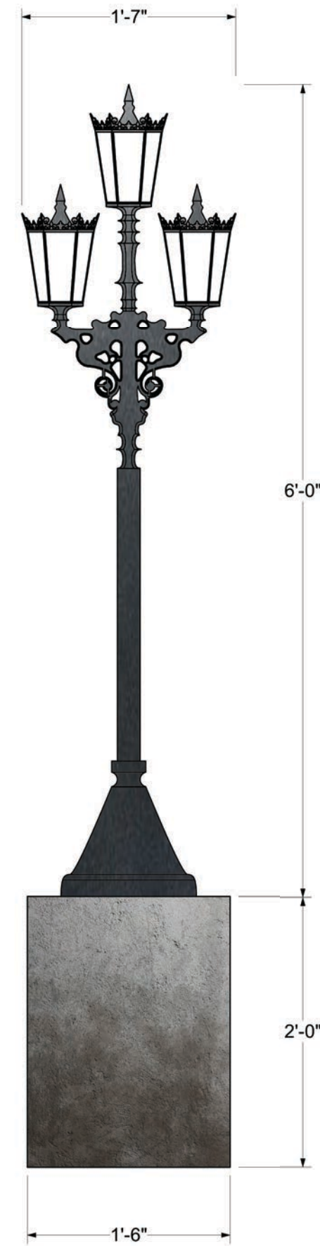
HAVANA STREETLIGHT SCALE: 1" = 1'-0" QTY: 3
